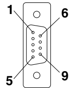
CN-2 (côté D-Sub 9 broches)
